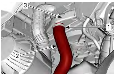
PASSAGE DE ROUE ARRIÈRE GAUCHE
