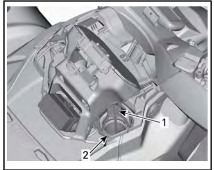
1. Filtro de aire de la CVT 2. Pestaña
