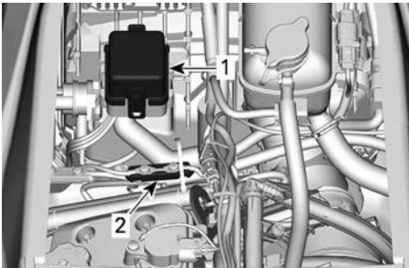
1. Zekeringskast 2. Hoofdzekering
