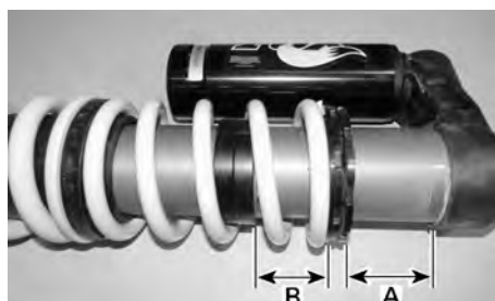
SITUAZIONE TIPICA - REGOLAZIONE CROSSOVER - AMMORTIZZATORE POSTERIORE
