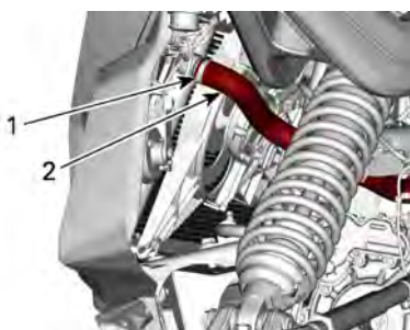
TUBO FLESSIBILE SUPERIORE DEL RADIATORE
