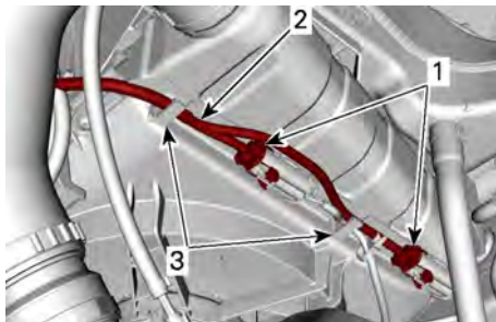
PASSAGE DE ROUE ARRIÈRE DROITE
