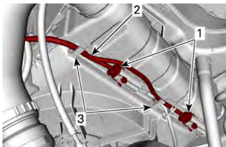
右后轮窝
