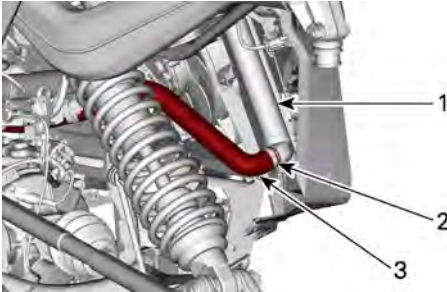
TUBO TUBO FLESSIBILE INFERIORE DEL RADIATORE
