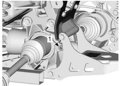
TRANSMISIÓN FINAL TRASERA, PARTE TRASERA IZQUIERDA DEL VEHÍCULO
