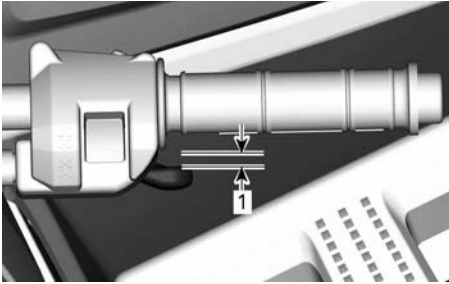
1. Gasfrispel
