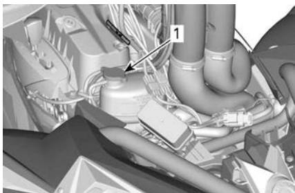
1. Dop motorkoelvloeistoftank
