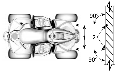
1. Middellijnen van koplamp
