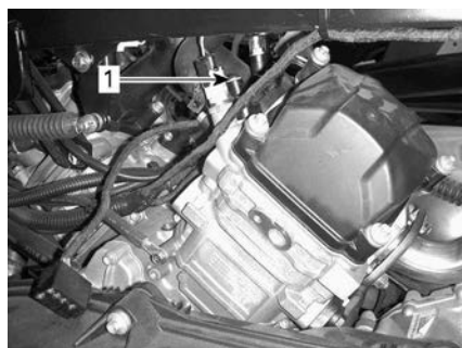
1. Vite di spurgo del cilindro posteriore
