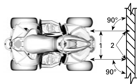
1. 大灯中心线
