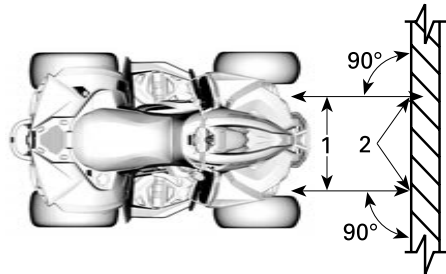
1. Líneas centrales del faro
