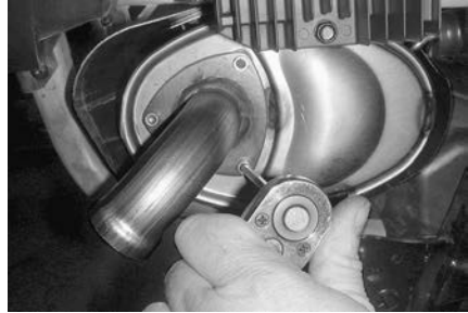
典型示例 - 拆卸尾管
