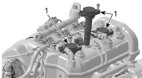
1. 点火线圈
