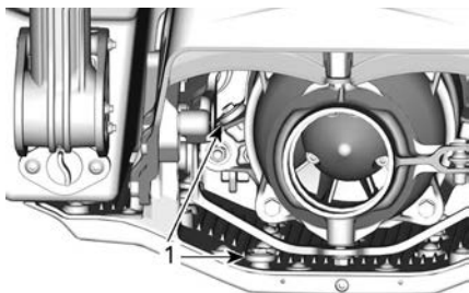
1. 牺牲阳极
