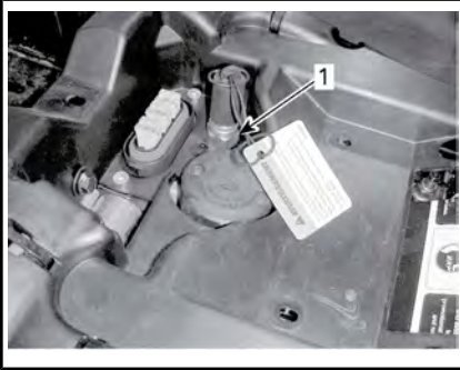
1. Kompressor-Anschlussstück
