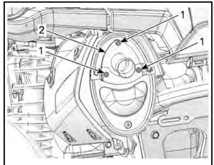
TYPISCH - ABGASROHR ENTFERNEN
