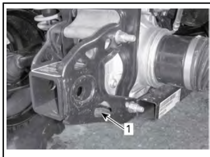
1. Hinterer Verzurtpunkt
