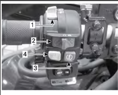
TYPISCH — MULTIFUNKTIONSSCHALTER
