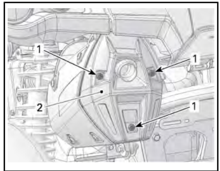
1. Abdeckung des Auspufftopfs 2. Ritzel
