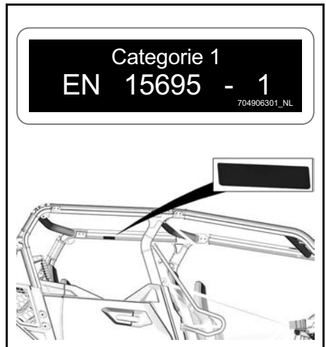
TYPISCH - NRMM-IDENTIFICATIELABEL
