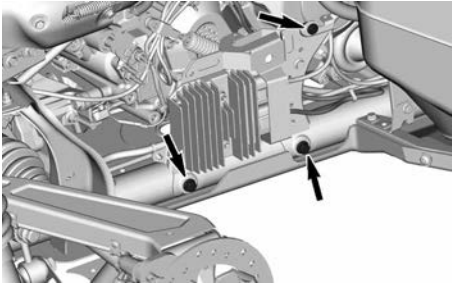
SCHROEVEN STEUN SPANNINGSREGELAAR
