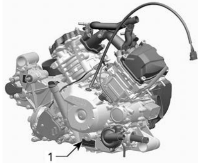
TYPBILD
