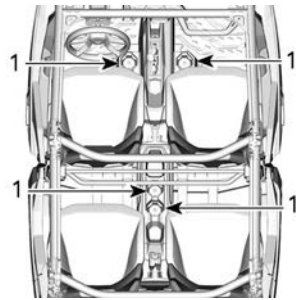
1. Sujetavasos
