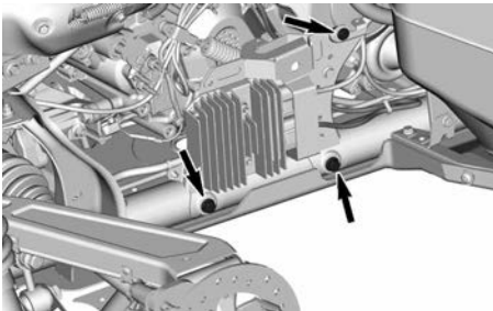
PARAFUSOS DE SUPORTE DA TENSÃO/ REGULADOR
