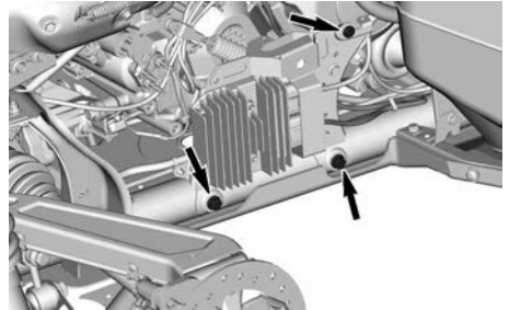
电压/调节器支架螺钉
