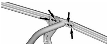
PARTE INFERIOR DO PILAR FRONTAL
