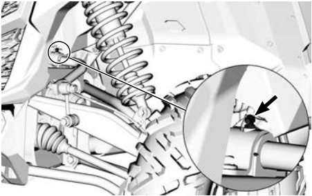
TÍPICO — BARRA ESTABILIZADORA DIANTEIRA
