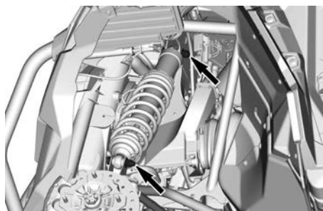
TÍPICO — FIXADORES DO AMORTECEDOR DIANTEIRO
