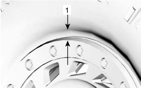
1. Folga igual em toda a volta do anel de aperto da trava de talão
