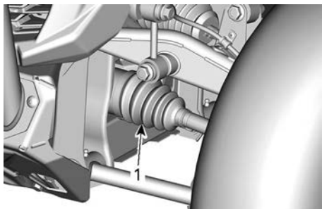
典型示例 - 前差速器侧
