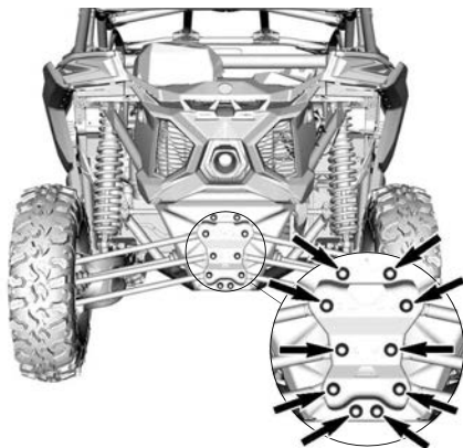
TYPIQUE - BARRE STABILISATRICE ARRIÈRE
