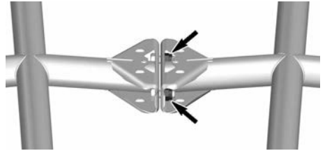
DISPOSITIVI DI FISSAGGIO CENTRALI
