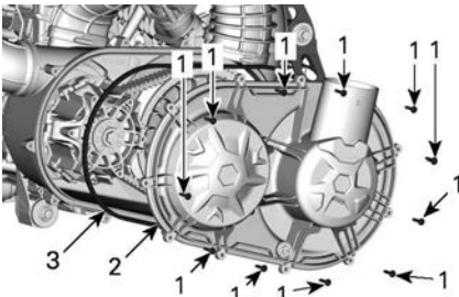
ILLUSTRATO MOTORE TURBO
