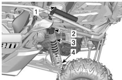
SITUAZIONE TIPICA - CON SMORZAMENTO IN ESTENSIONE E SERBATOIO REMOTO - SOSPENSIONE POSTERIORE
