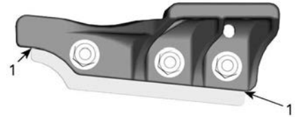
1. Limite di usura
