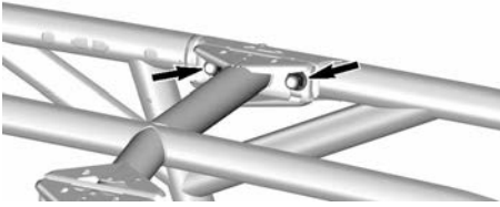
MITTLERE, BEFESTIGUNGSELEMENTE OBERE
