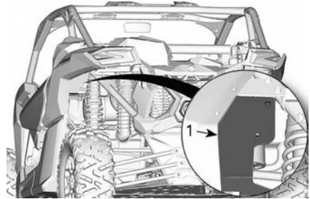
1. Beskyttelsesplate
