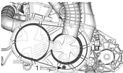
1. CVT-avløp
