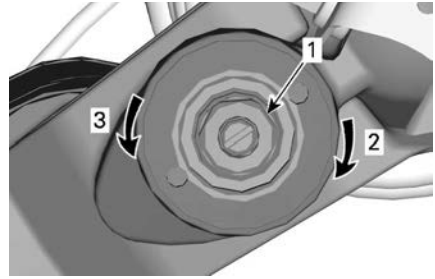
SMORZAMENTO IN COMPRESSIONE AD ALTE VELOCITÀ (UTILIZZARE UNA CHIAVE INGLESE DA 17 MM)
