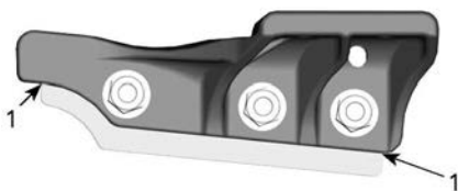
1. Limite d'usure
