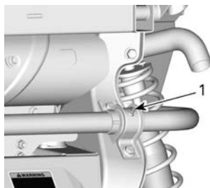
典型示例 1. 后平衡杆衬套黄油嘴
