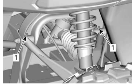
1. Fjädringsarmens smörjnipllar
