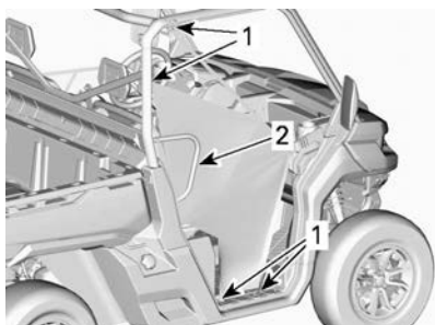
1. Justeringsplatser för sidonätet 2. Axelskydd
