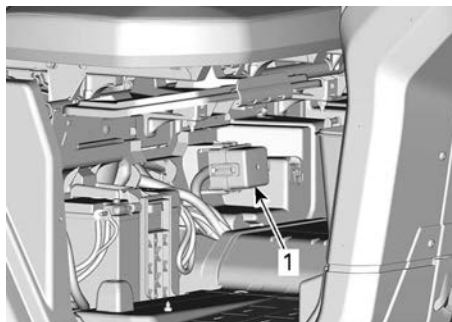
1. Toissijainen takasulakelaatikko
