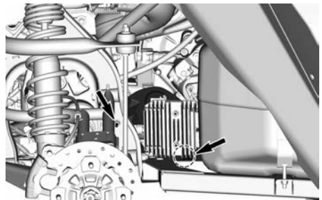
UBICACIÓN DE LAS SUJECIONES DEL SOPORTE DEL REGULADOR DE VOLTAJE
