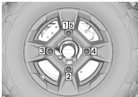
SECUENCIA DE APRIETE
