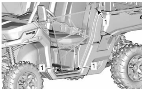
1. Ubicaciones de ajuste de las redes laterales
