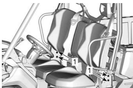
1. Fixations inférieures de la cage
