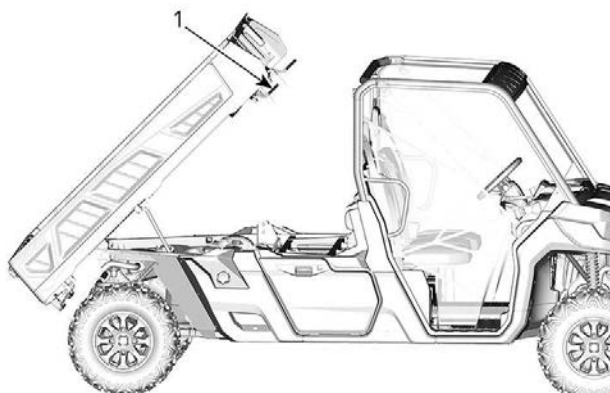
1. Spärrhandtag
