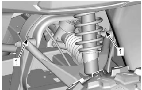
1. Sospensioni - punti di ingrassaggio braccio
