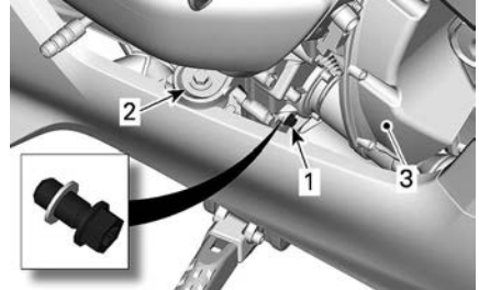
VAIHTEISTOÖLJYN SIJAINTI
