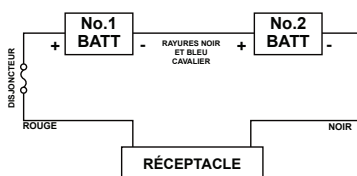
12/24V SYSTÈME DE PÊCHE A LA TRAÎNE
