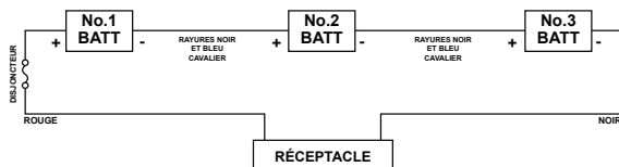
12/24/36V SYSTÈME DE PÊCHE A LA TRAÎNE
