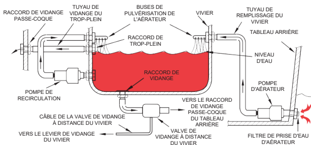
VIVIER AVEC VALVE DE VIDANGE À DISTANCE ET SYSTÈME DE RECIRCULATION
