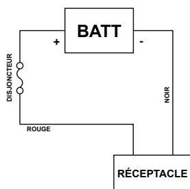
12V SYSTÈME DE PÊCHE A LA TRAÎNE
