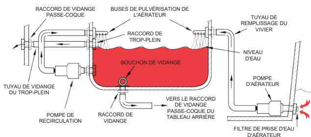
VIVIER AVEC BOUCHON DE VIDANGE, SYSTÈME DE VIDANGE ET SYSTÈME DE RECIRCULATION
