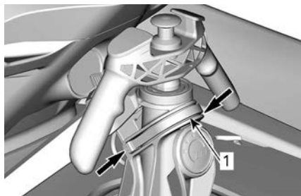
代表的な例 - パイロンを前方に押し、ロッキングクリップを解除し、取り外す
