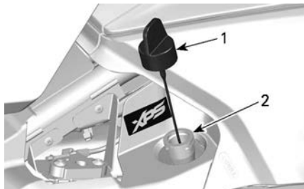
1. Jauge de niveau d'huile 2. Tube de remplissage d'huile
