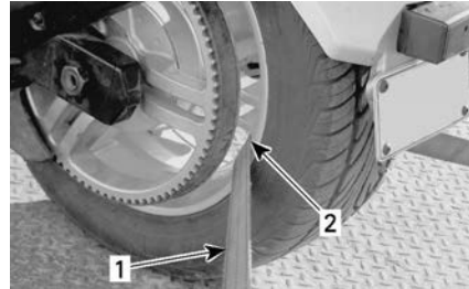
ARRIMAGE DE LA ROUE ARRIÈRE — TYPIQUE
