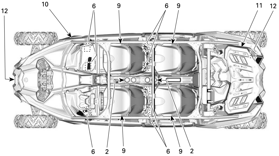
TÍPICA – MAVERICK MAX (SUPERIOR)
