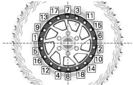
TYPISCH - AANDRAAIVOLGORDE
