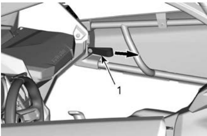
1. Vergrendelband
