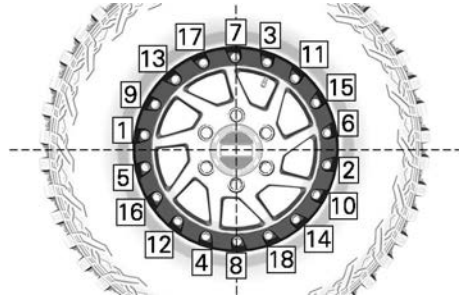
TYPISCH - AANDRAAIVOLGORDE
