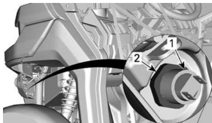
1. Luci di posizione 2. Dadi di fissaggio
