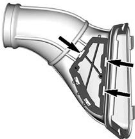
6. Ta bort CVT-luftfiltret.
