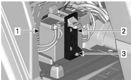
1. Batterie 2. Support de batterie 3. Vis de fixation du support de batterie.
