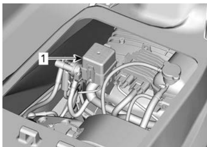
1. Scatola fusibili
