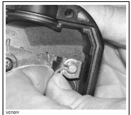
6. Irrota kaasuläppärungon sivukansi.
