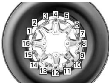
TYPBILD - SLUTLIG ÅTDRAGNINGSEKVEN
