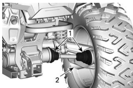
典型示例 - 车辆后部
