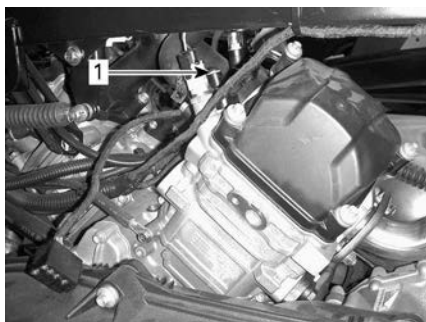
1. 后气缸放气螺钉
