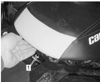
1. 座椅锁扣
